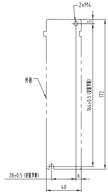
安装孔加工图
