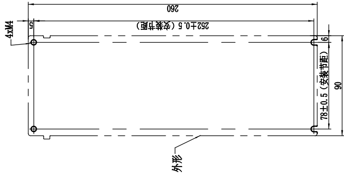
安装孔加工图 单位: mm
