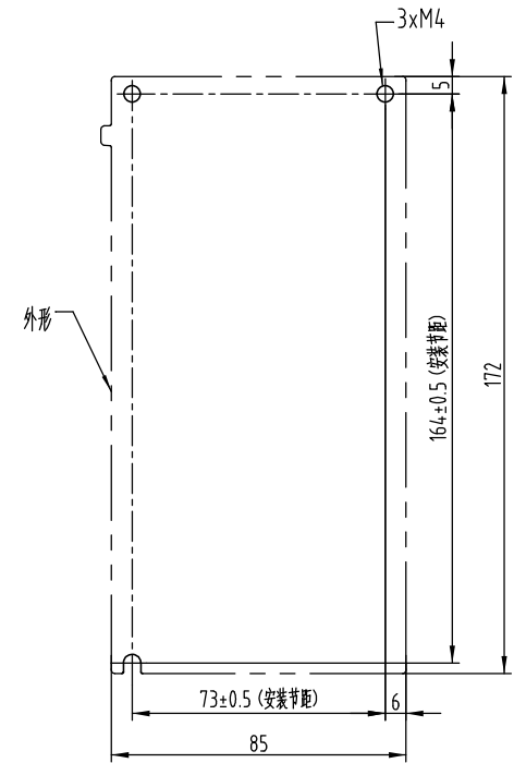
安装孔加工图
