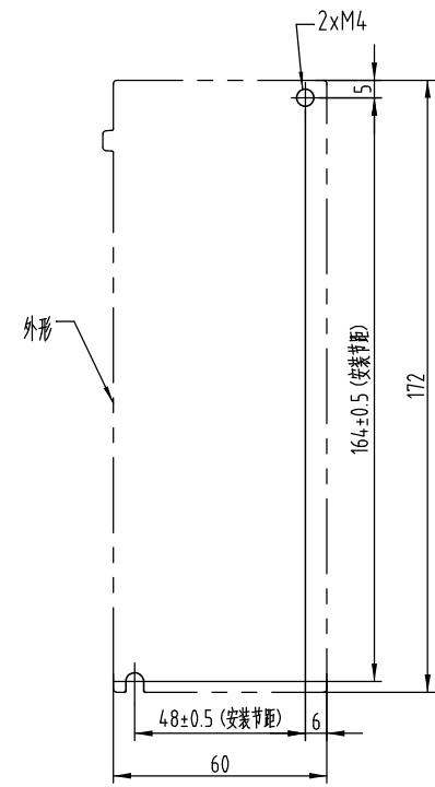
安装孔加工图 单位: mm
