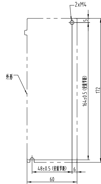
安装孔加工图 单位: mm
