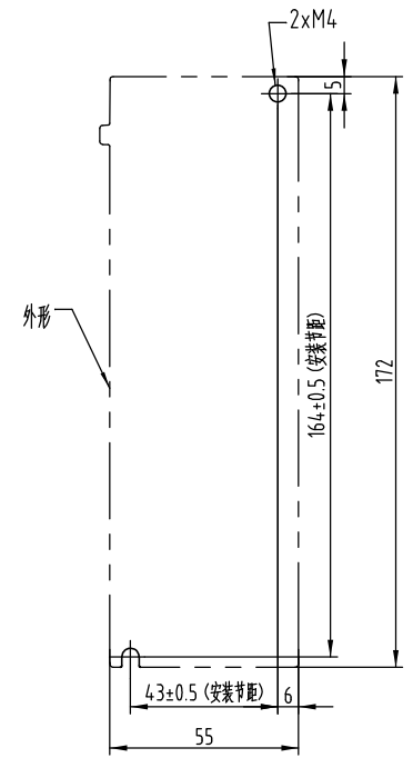
安装孔加工图
